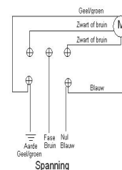
Aansluitschema Pisto en Geba Schakelaar
